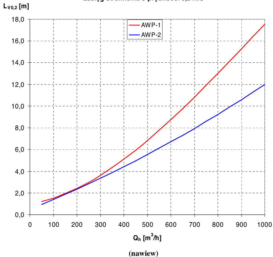
Zasięg strumienia o prędkości 0,2 m/s
