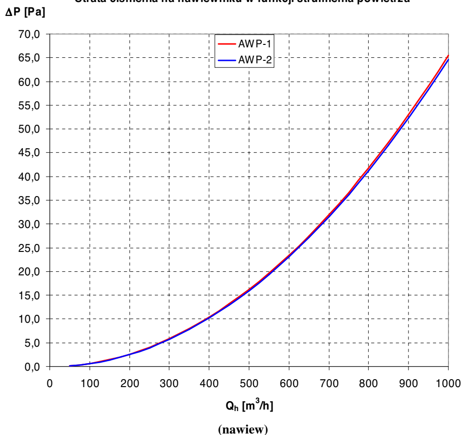
Strata ciśnienia na nawiewniku w funkcji strumienia powietrza
